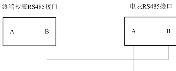
图 6 RS485 抄表接线
