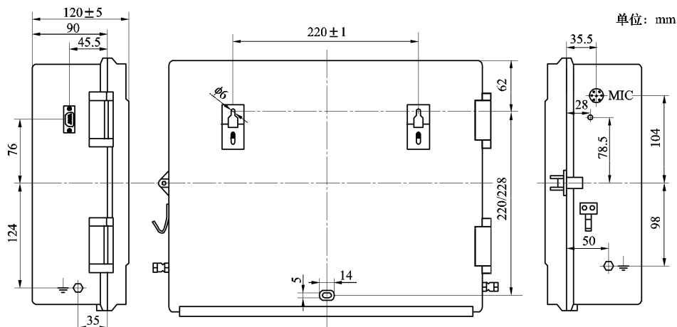
图2 终端尺寸图
