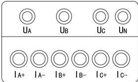
图 4-1 交采输入端子图
