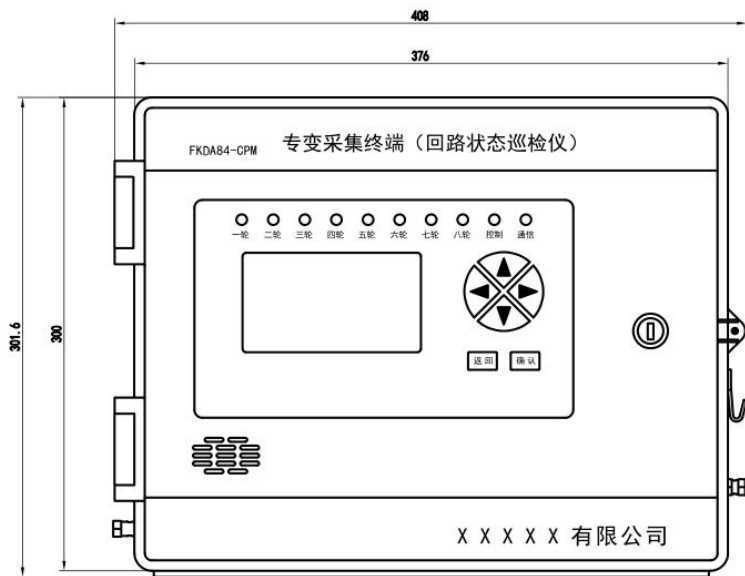
图 1 终端面板图
